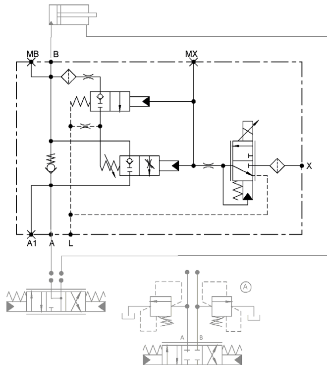
Schaltschema elektrisch
