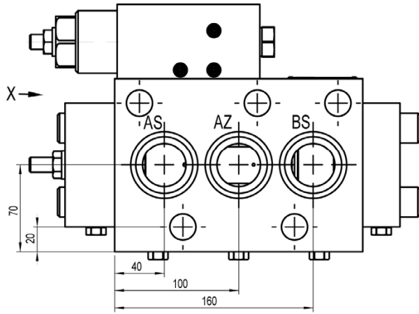
800 l/min Version links (rechte Version gespiegelt)
