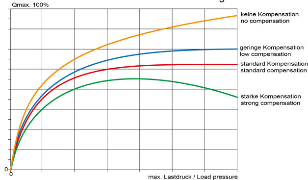
Durchflusskennlinie für maximales Vorsteuersignal
