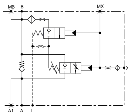
Schaltschema hydraulisch
